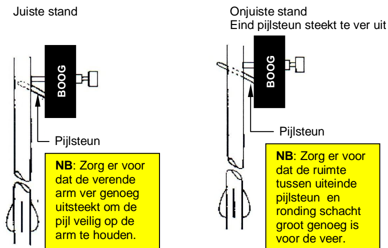
Figuur 8 Bovenaanzicht pijlsteun (RF, CF)
